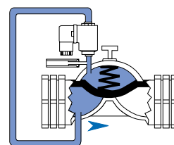
VALVULA CERRADA
